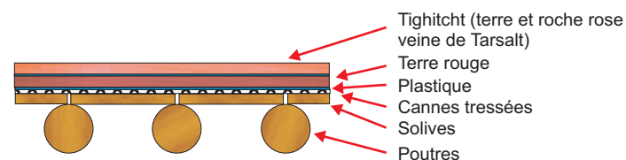
Technique de la couverture traditionnelle
